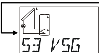
Volumenstromgeber (Impulsgeber)
