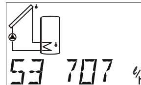
Durchfluss in l/h (Sensor 3 = VFS 2-40)
