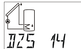
Drehzahlstufe nur bei ESR31-D und aktiver PDR
