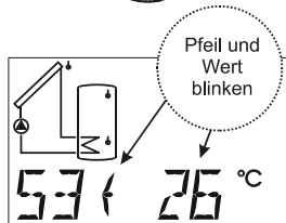
Fixwert Eingabe
