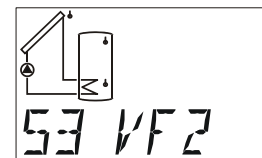
Vortex – Sensor Volumen 2-40l/min
