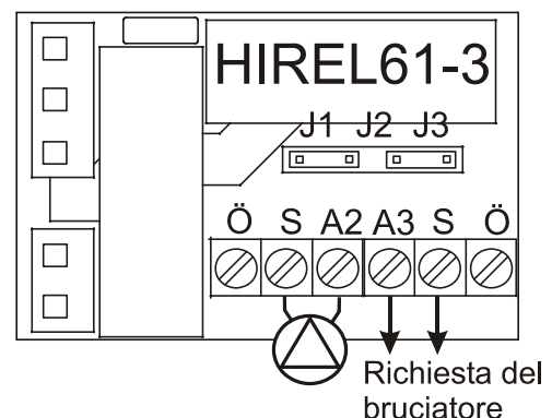
Schema 16: Collegamento di una pompa su A2 e della richiesta della caldaia su A3 (se necessario azionare senza tensione):
