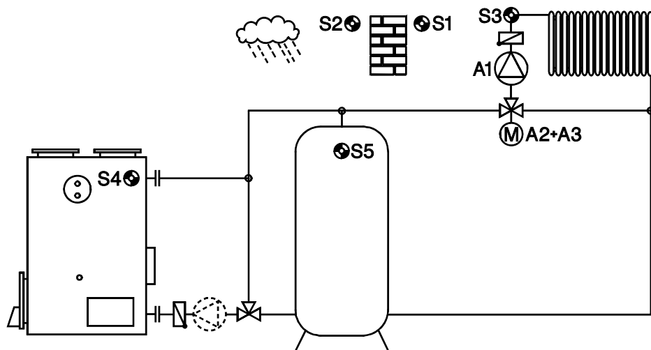
Schema 0: Circuito di riscaldamento con fino a 2 fonti di calore
