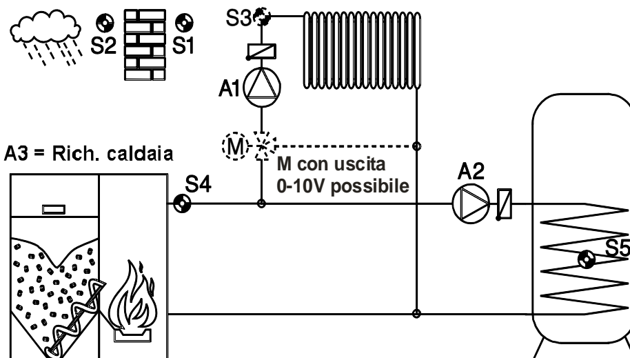
Schema 16: Caldaia automatica, boiler, circuito di riscaldamento (senza miscelatore), richiesta caldaia
