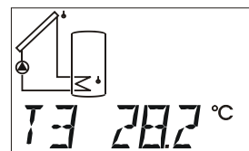
Teplota čidlo 3
