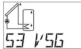
Emisor de caudal (emisor de impulsos) (sólo sensor S3)
