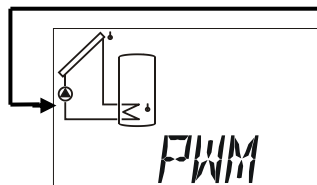
Sortie PWM
