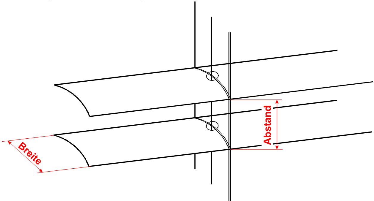
• Abbildung 1: Lamellenabmessungen
