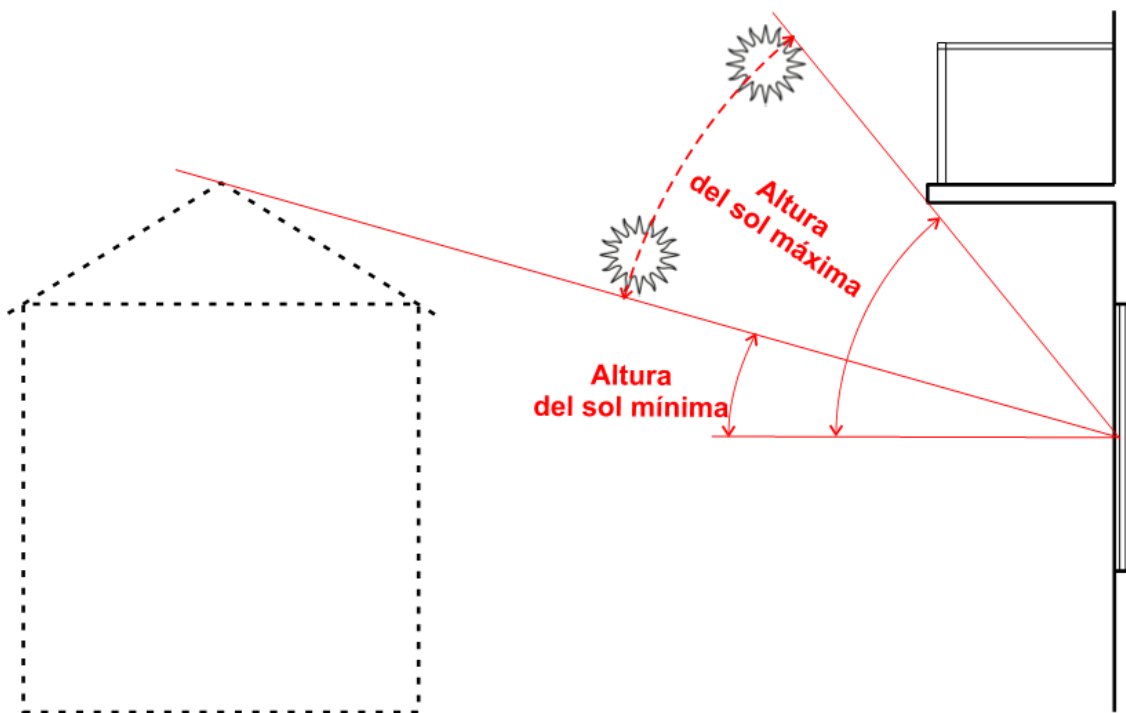
• Figura 3: Altura máxima y mínima del sol (ilustración: proyección vertical)
