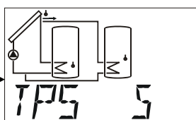
Tiempo de espera en la prioridad subsiguiente
