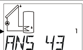
Stopień analogowy wyświetlany tylko wtedy, gdy aktywne jest wyjście sterujące
