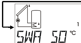
Wartość zadana dla regulacji wartości bezwzględnej
