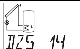
Stopień prędkości obrotowej wyświetlany tylko wtedy, gdy aktywna jest regulacja prędkości obrotowej
