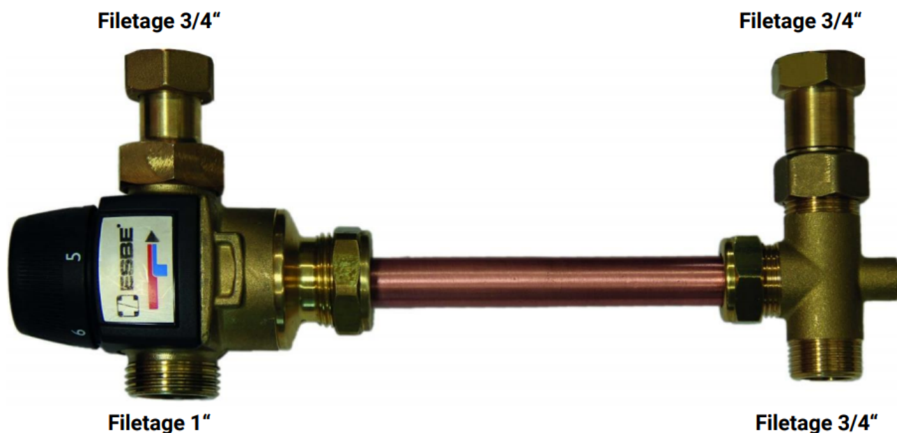
Figure : raccordement pour FRISTAR avec pompe à droite
