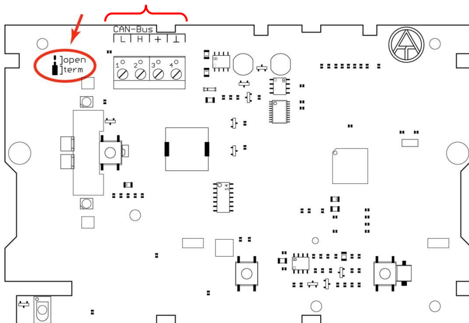
Terminazione Collegamento CAN-Bus
