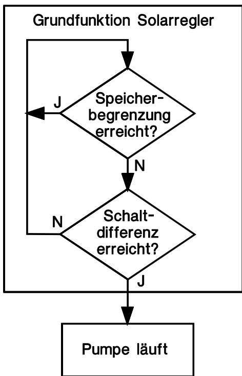
Einfacher Solarregler
